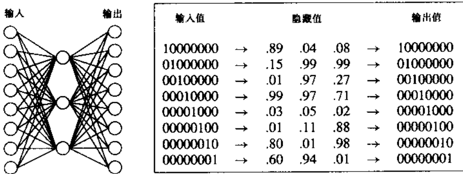
这个 8 \times 3 \times 8 的网络被训练以学习恒等函数，使用图中所示的 8 个训练样例。在 5000 轮(epochs)训练之后，3 个隐藏单元使用图右侧的编码方式来编码 8 个相互不同的输入。注意，如果把编码后的值四舍五入为 0 和 1，那么结果是 8 个不同值的标准二进制编码
