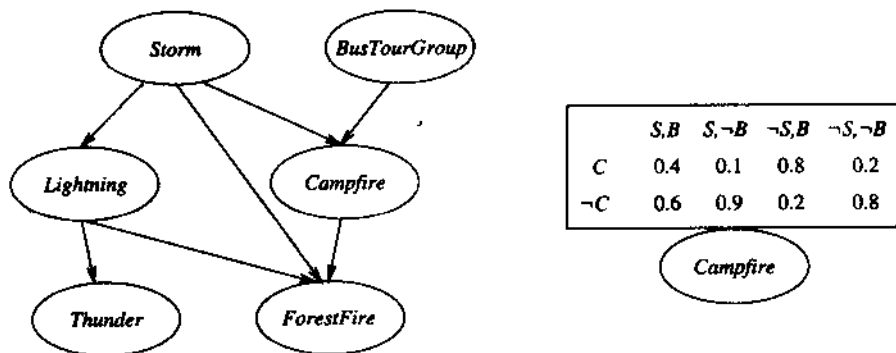
左边的网络表示了一组条件独立性假定。确切地说,每个节点在给定其父结点时,条件独立于其非后代结点。每个结点关联一个条件概率表,它指定了该变量在给定其父结点时的条件分布。右边列出了 Campfire 结点的条件概率表,其中 Campfire 、 Storm 和 BusTourGroup 分别缩写为 C, S, B
