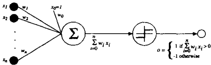
图 4-2 感知器
