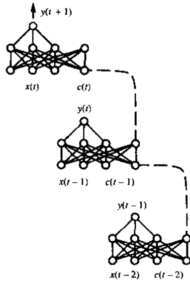
图 4-11 递归网络
