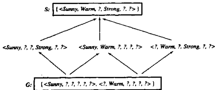
变型空间中包含了所有 6 个假设,但可以简单地用 S 和 G 来表示。箭头表示实例间的 more_general_than 关系。这个变型空间对应于表 2-1 中描述的 EnjoySport 概念学习问题及其训练样例
