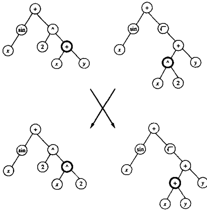
双亲程序树显示在上方,孩子树在下方。交叉点(上边加粗显示的节点)是随机选取的。然后以这些交叉点为根的子树互换以产生孩子树
