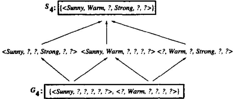
图 2-7 EnjoySport 概念学习问题中的最终的变型空间
