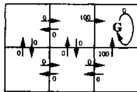
r(s, a) 立即回报值
