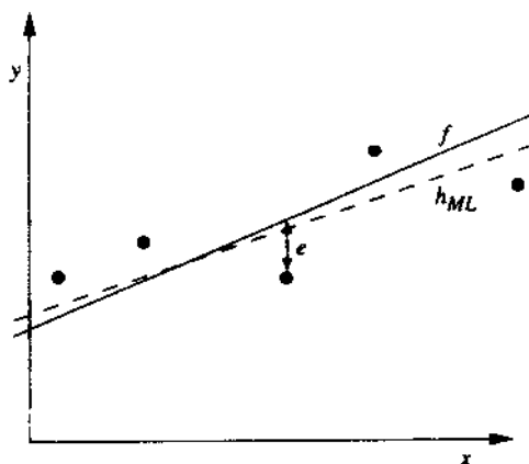
目标函数 f 对应实线。假定训练样例 \langle x_i, d_i \rangle 为真实目标值加上一零均值的正态分布噪声 e_i 。虚线代表使误差平方之和最小的线性函数。因此,它就是这 5 个训练样例下的极大似然假设 h_{ML}
