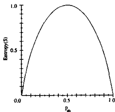
图中画出了随着正例所占比例 p_{\oplus} 从 0 到 1，熵函数变化的曲线
