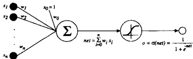
图 4-6 sigmoid 阈值单元
