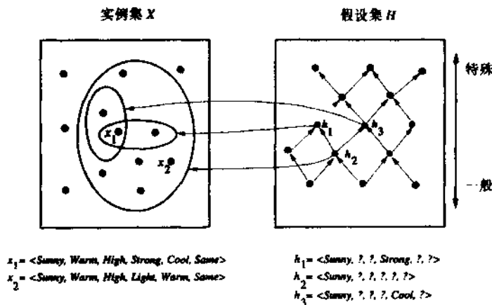
左边的方框代表所有实例的集合 X ，右边的方框代表所有假设集合 H 。右边的每个假设对应左边 X 中某个子集——即被此假设划分为正例的集合。连接假设的箭头代表 more_general_than 关系。箭头所指为较特殊的假设。注意到 h_2 对应的实例子集包含了 h_1 对应的实例子集，因此 h_2 more_general_than h_1 。
